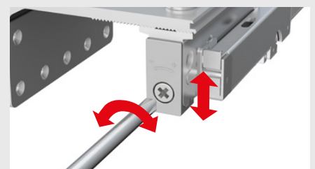
Regolazione verticale post-montaggio dell'anta. Door vertical adjustment.
